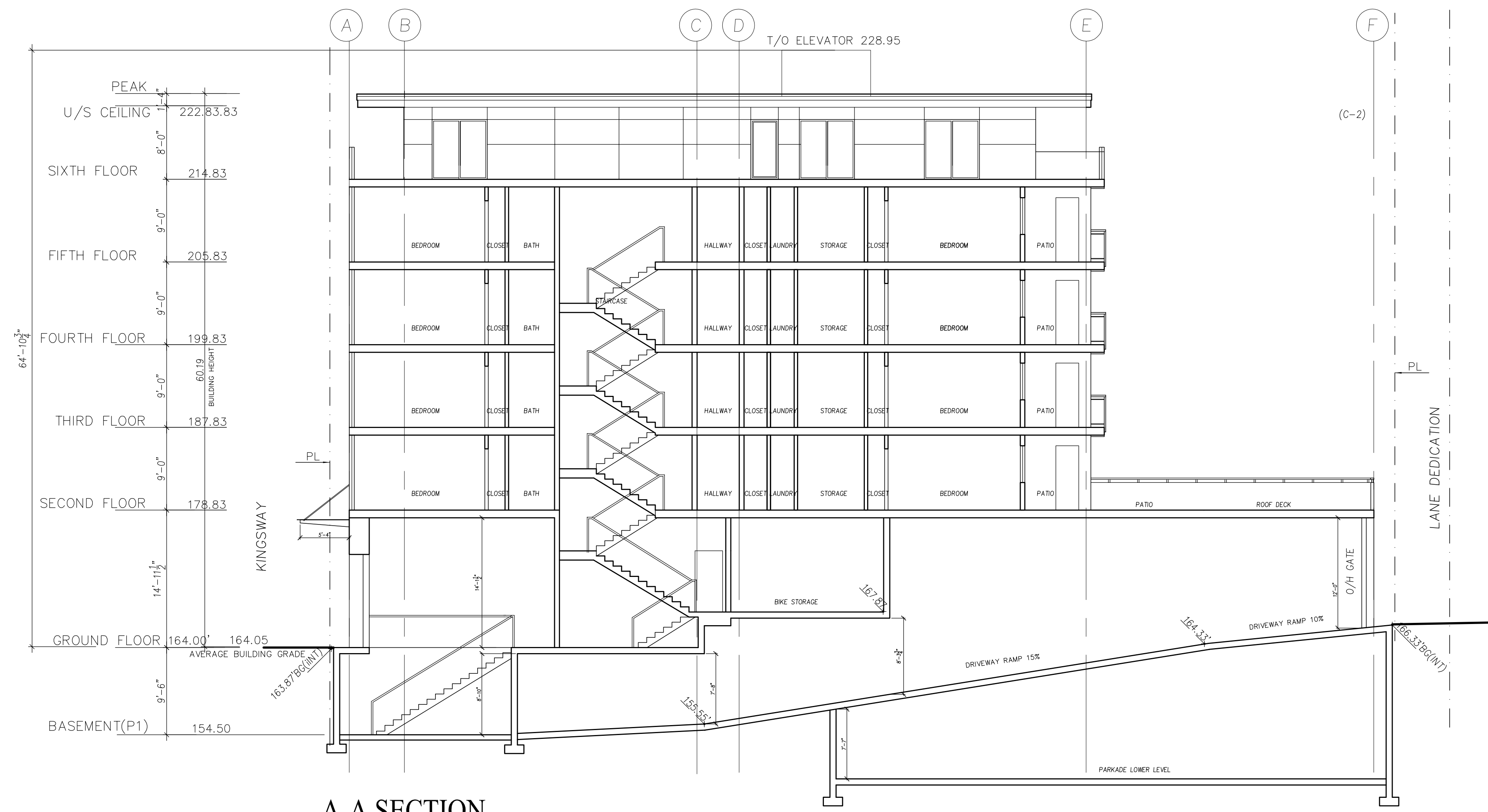
A-A SECTION
