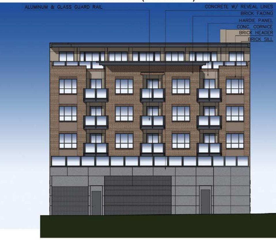
EAST ELEVATION (LANE)
