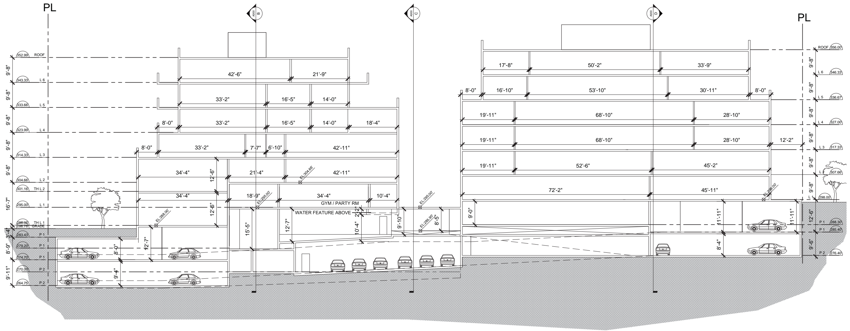
SECTION A-A
