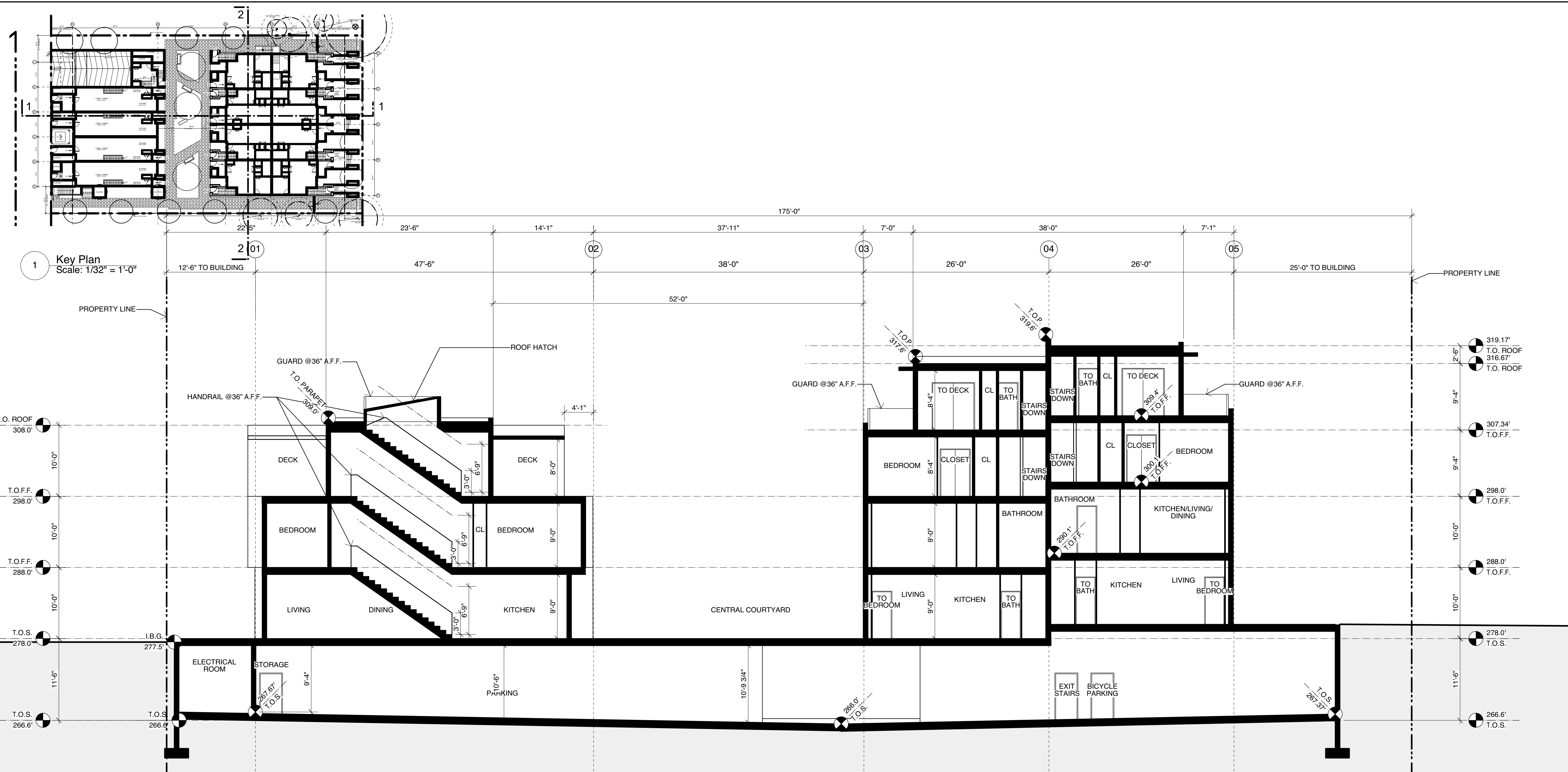
2 Section 1-1 Scale: 1/8" = 1'-0"
