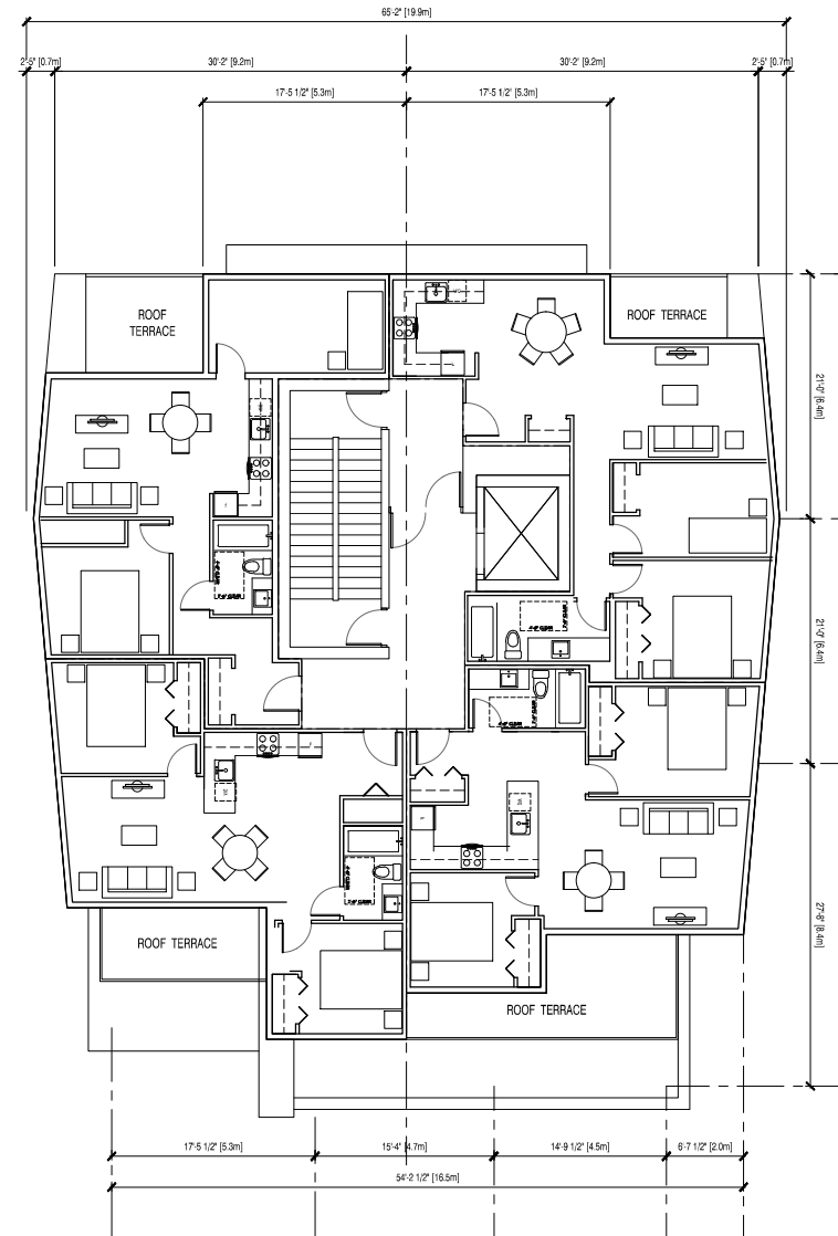
3 Level 6 Plan SCALE: 1/8" = 1'-0"
