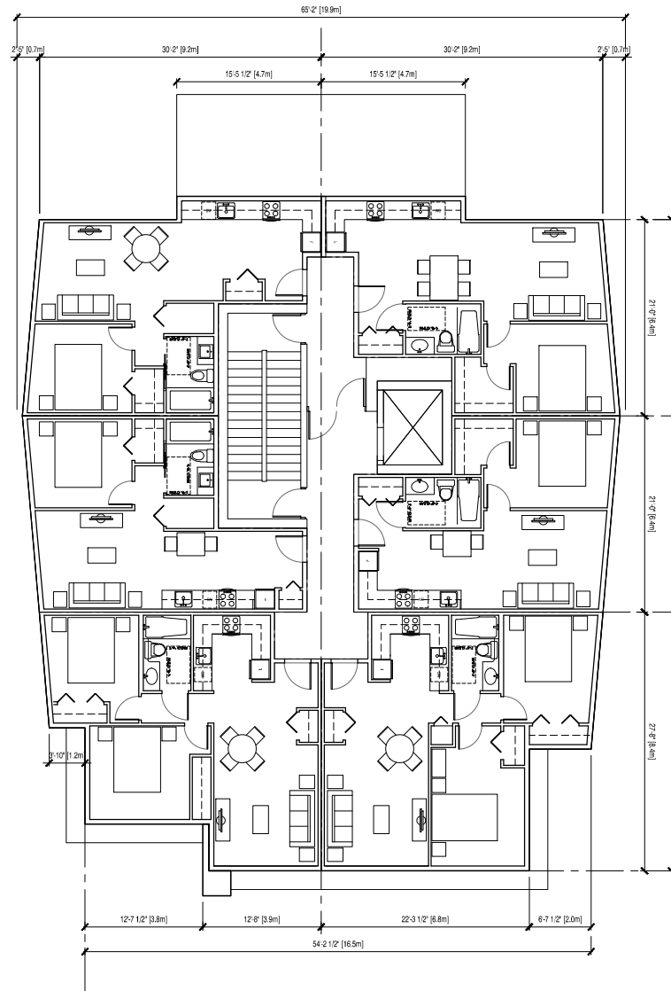
1 Level 3 Plan SCALE: 1/8" = 1'-0"
