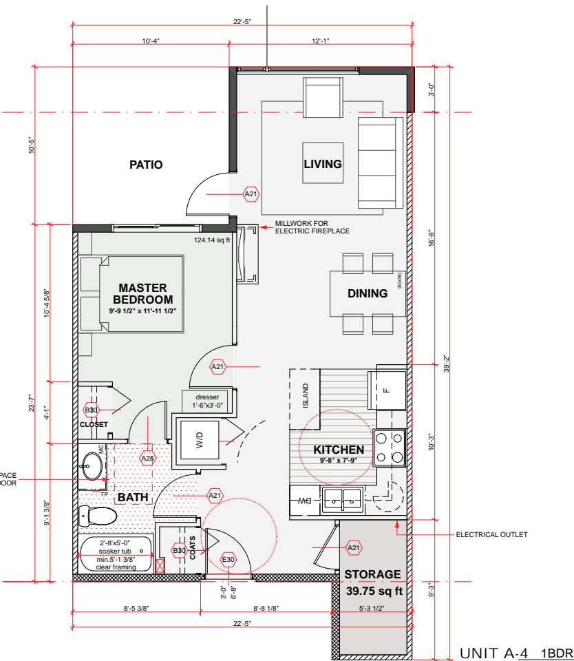
UNIT A-4 1BDRM 682.38 sq ft
