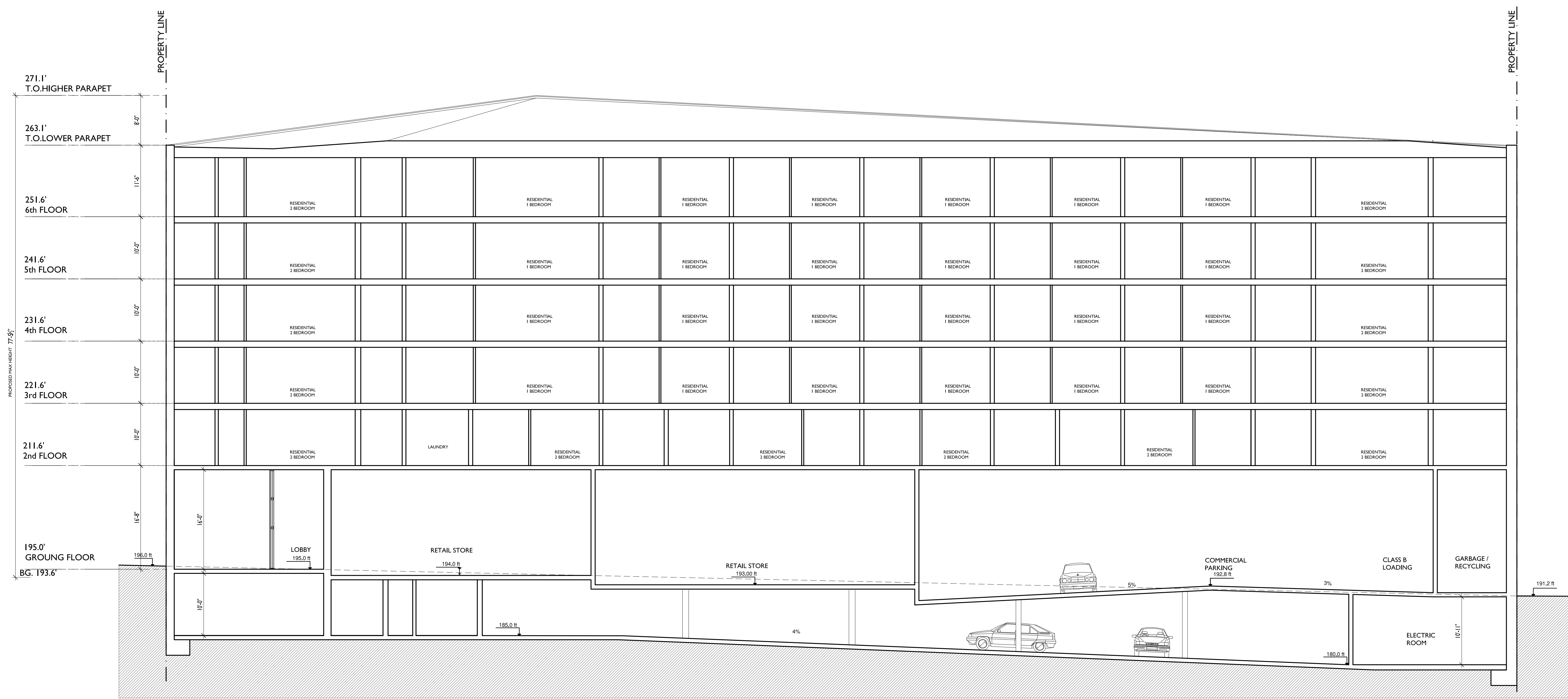
SECTION A-A
