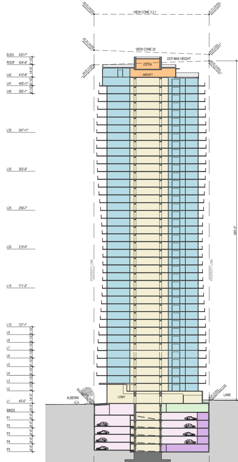
4.4.1 Section A A
