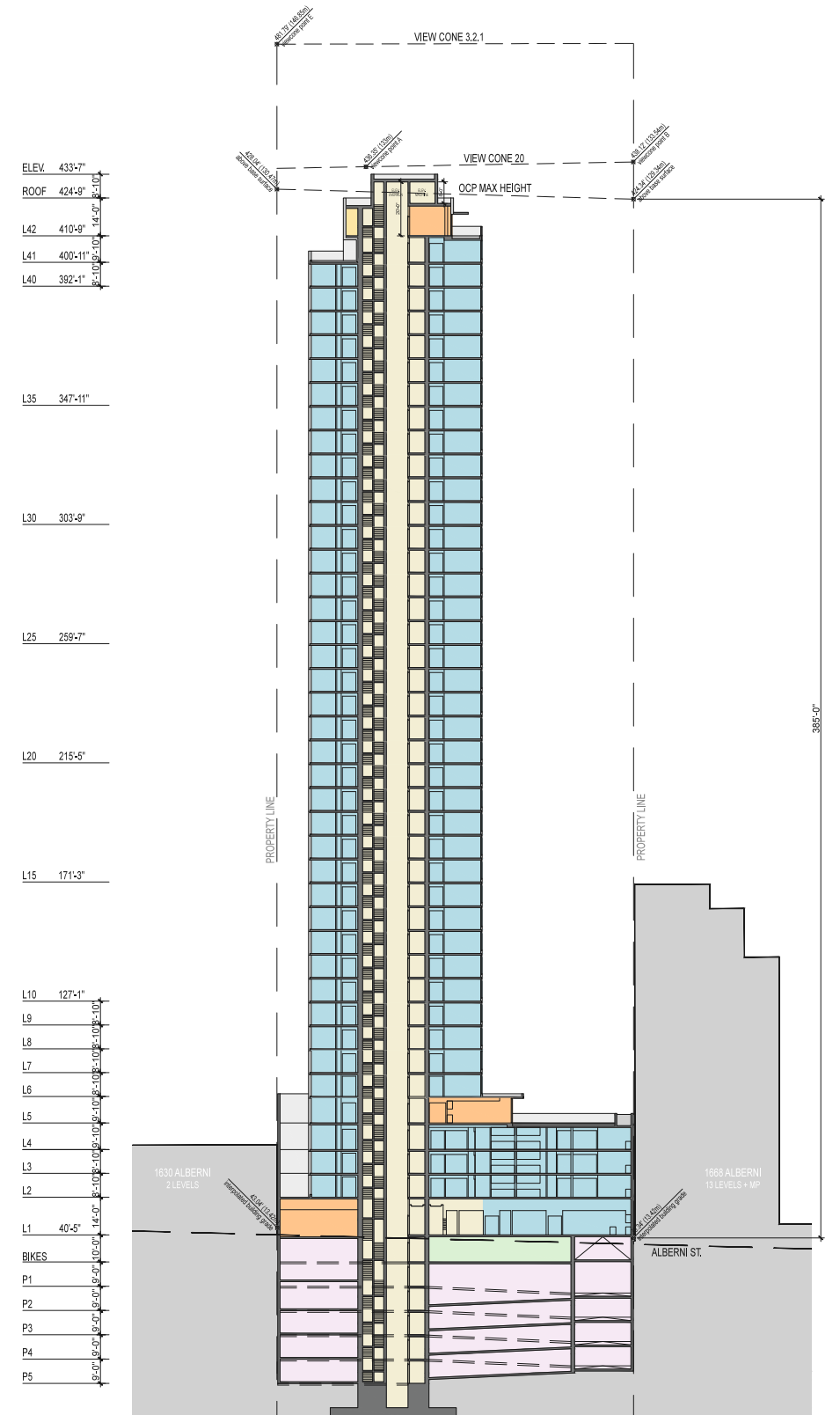
4.4.2 Section B B
